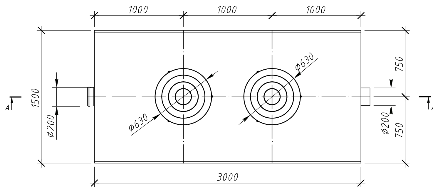
Вид сверху
