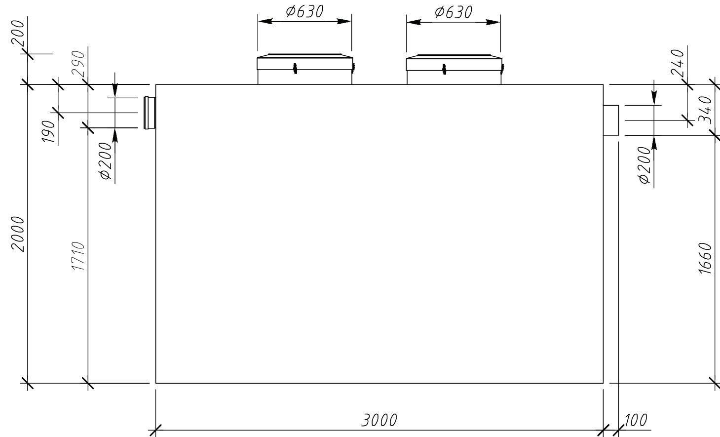
Вид спереди
