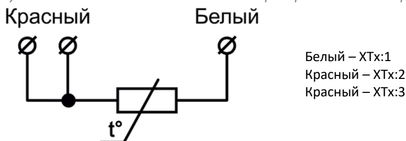
Рисунок 26. Схема подключения датчиков преобразователей термосопротивления серии ДТС 064.
