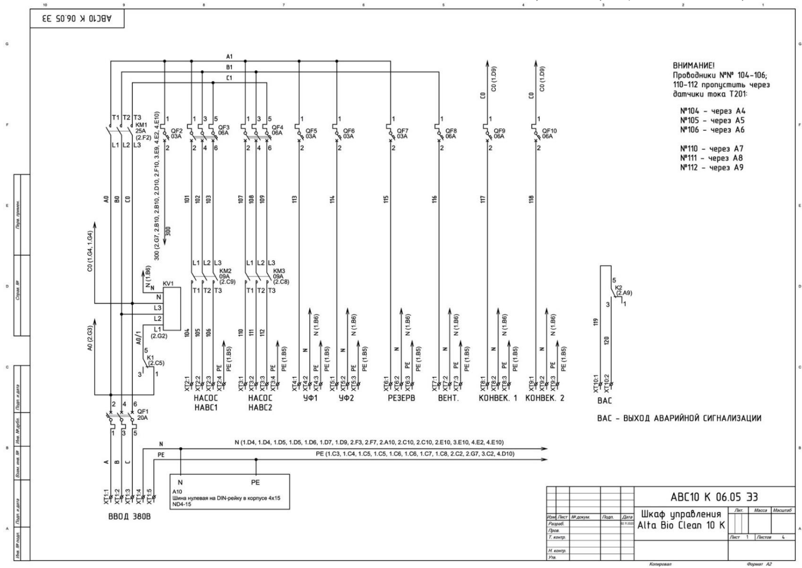
Рисунок 43. Принципиальная электрическая схема Блока.
