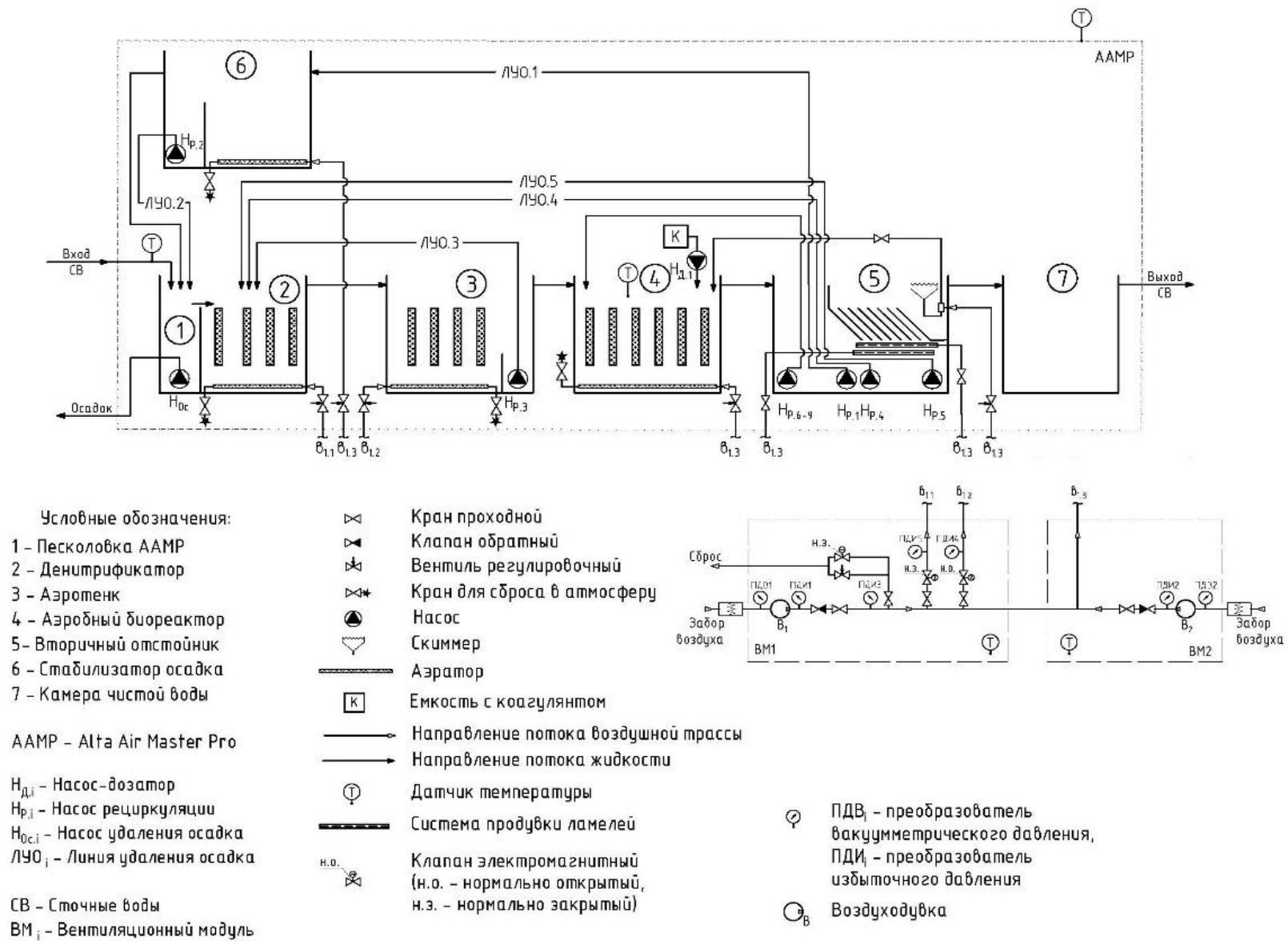
Рисунок 5. Технологическая схема Станции.
