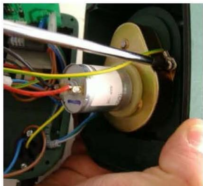
Рисунок 55. Порядок действий при замене прижимных роликов в насосе-дозаторе Etatron B3-V PER 1–3 90/260V SANT
