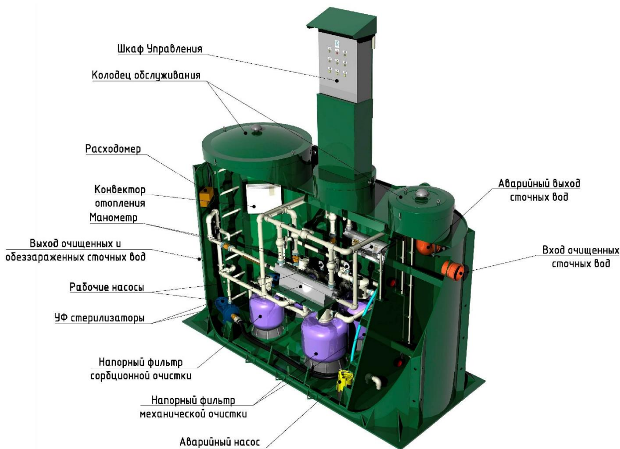
Рисунок 3. Пример компоновки Блока УФ обеззараживания Alta BioClean подземного монтажа
