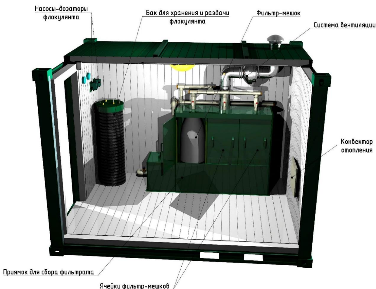
Рисунок 58. Пример исполнения обезвоживателя мешкового
