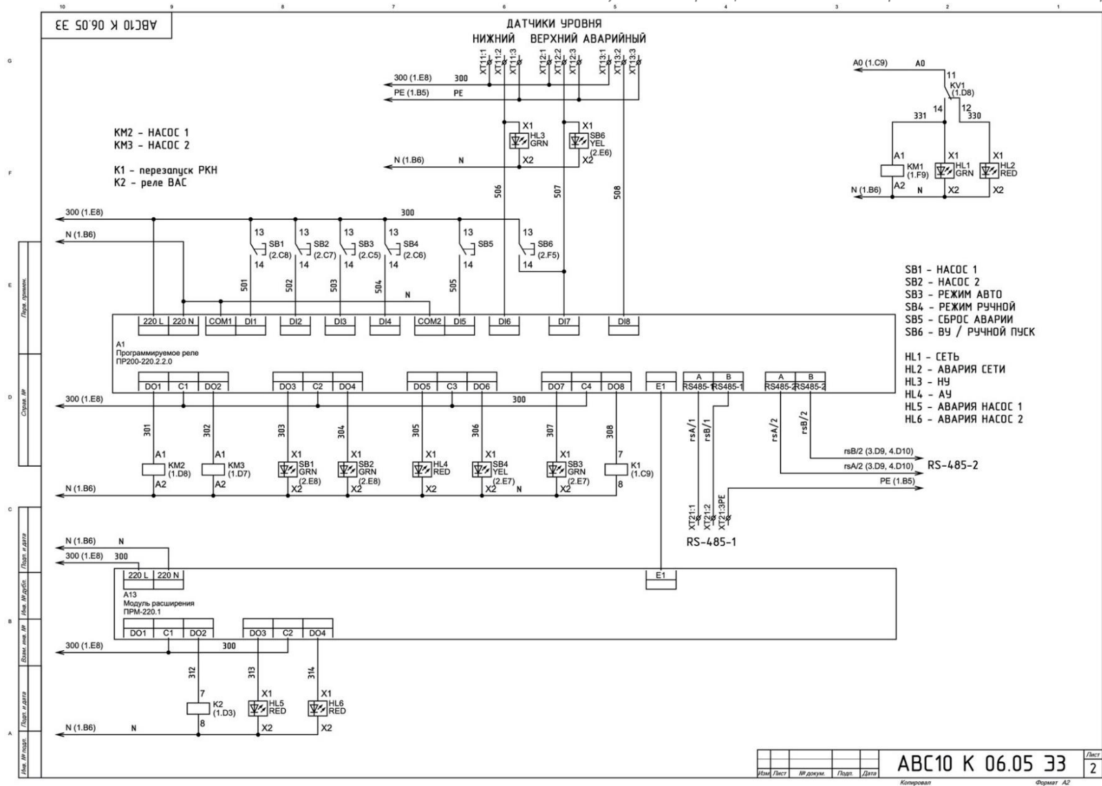
Рисунок 43. Принципиальная электрическая схема Блока. Продолжение.
