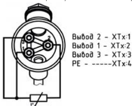
Рисунок 25. Схема подключения датчиков преобразователей термосопротивления серии ДТС 105.
