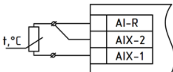
Рисунок 27. Схема подключения датчиков преобразователей термосопротивления по трехпроводной схеме.
