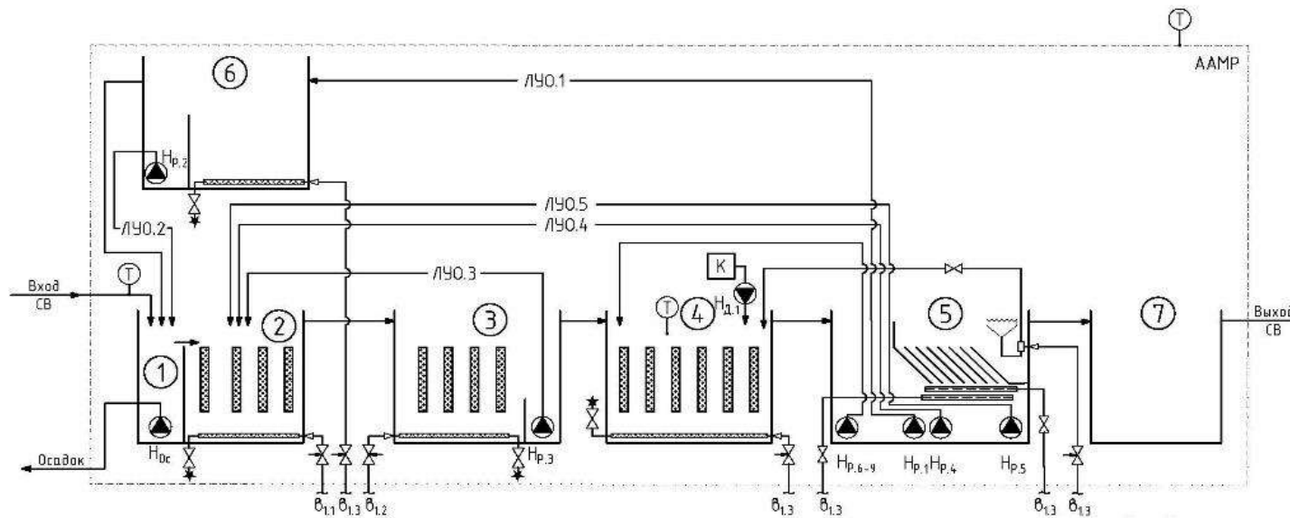
Рисунок 5. Технологическая схема Станции.
