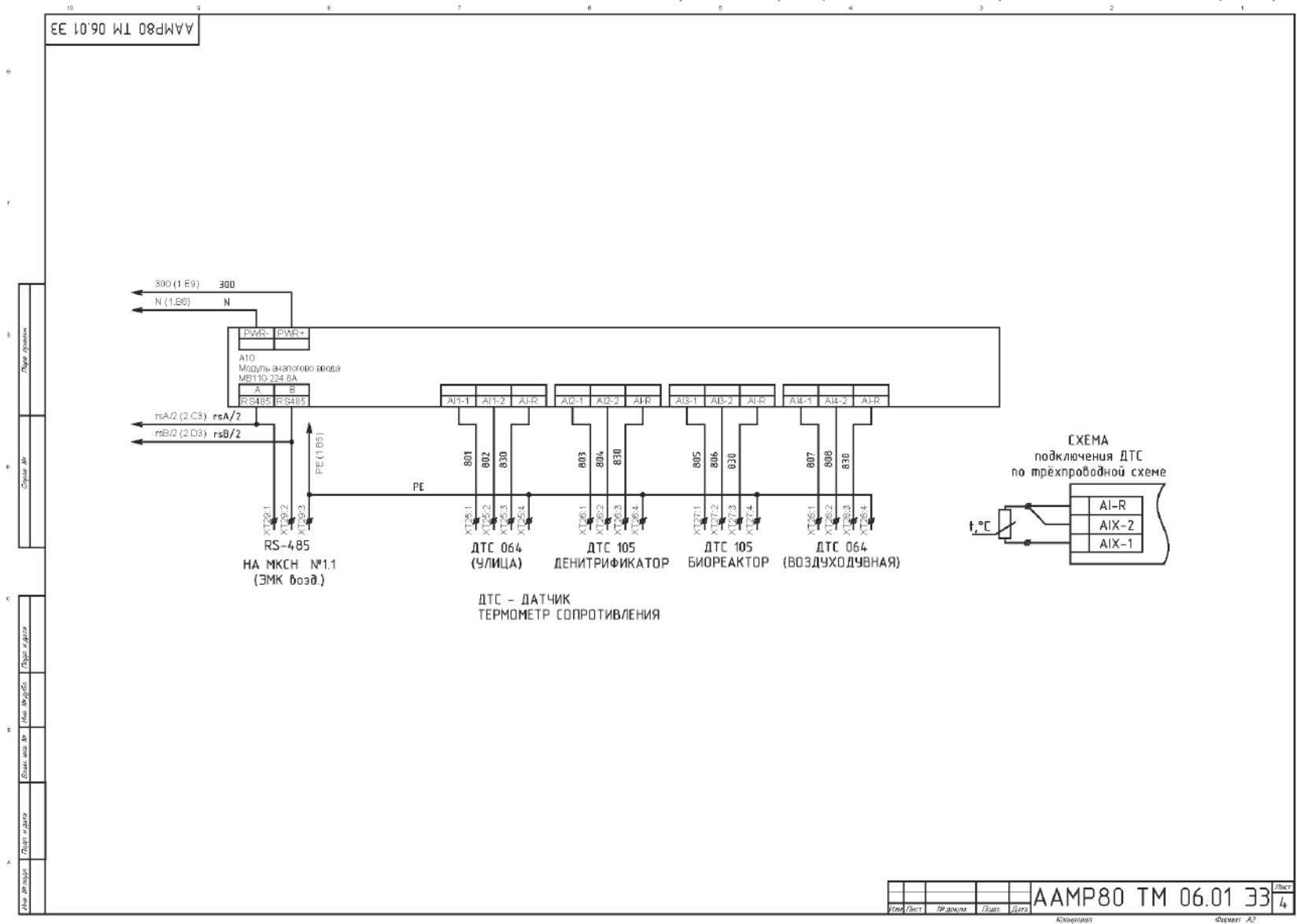
Рисунок 31. Принципиальная электрическая схема Станции. Продолжение.
